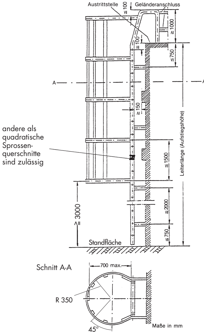
Bild 5: Steigleiter mit Rückenschutz
